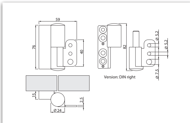
Dimensioning
