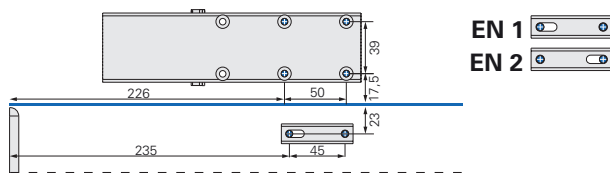
Closing force EN 1/2
